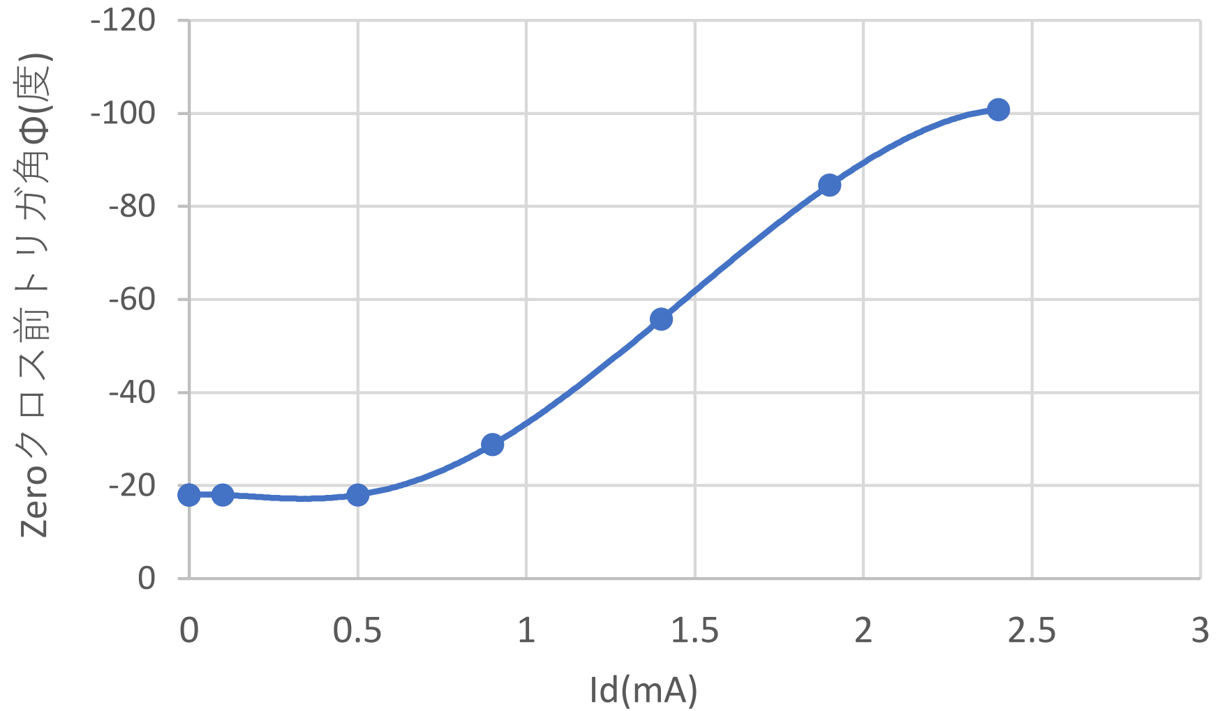
Diode電流 I_d とZeroクロス前トリガ角 \Phi
